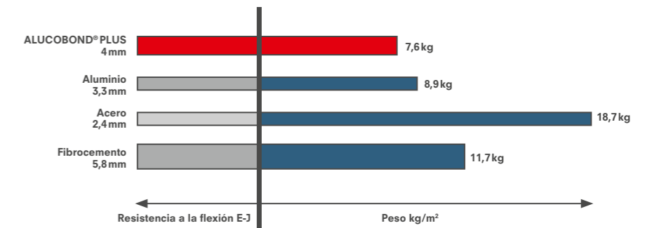
Comparación entre el grosor y el peso una misma rigidez
