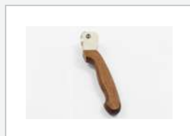
Cross-Cut Test Teste de aderência da pintura
